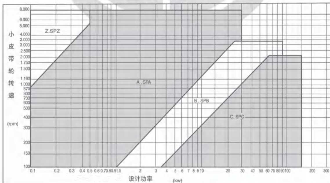
V型带皮带轮型号选用图
